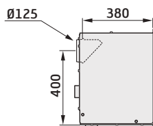
Conduit de fumée vers l'arrière Manchon Ø 125 mm
